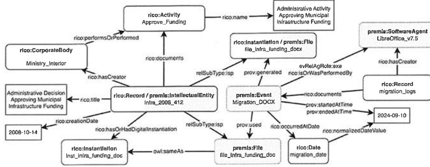
Fig. 1. Example - PREMIS & RiC-O.
